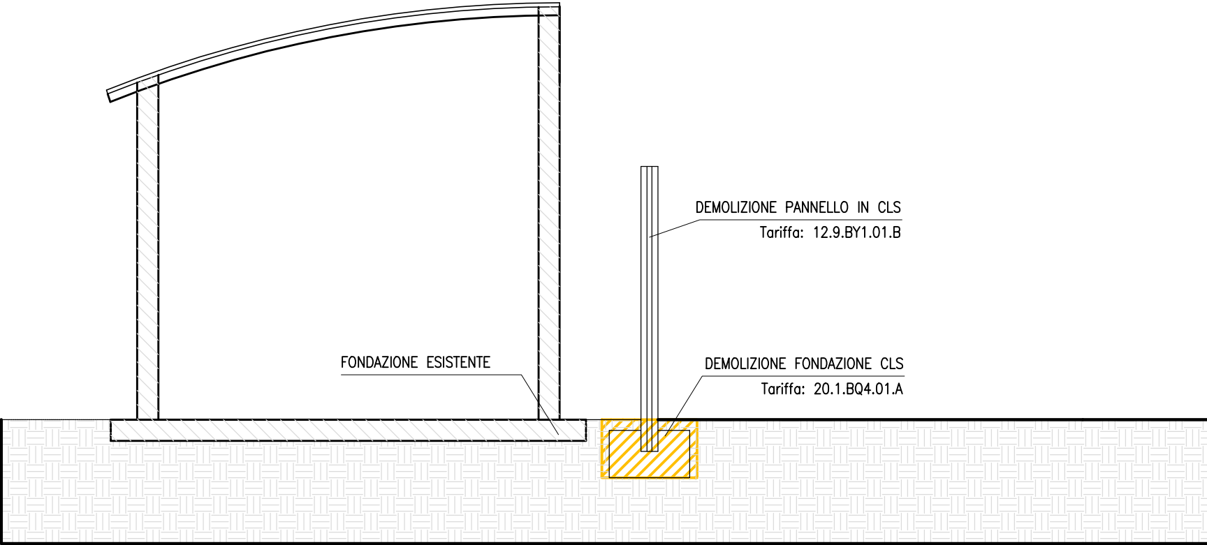
SEZIONE A-A
