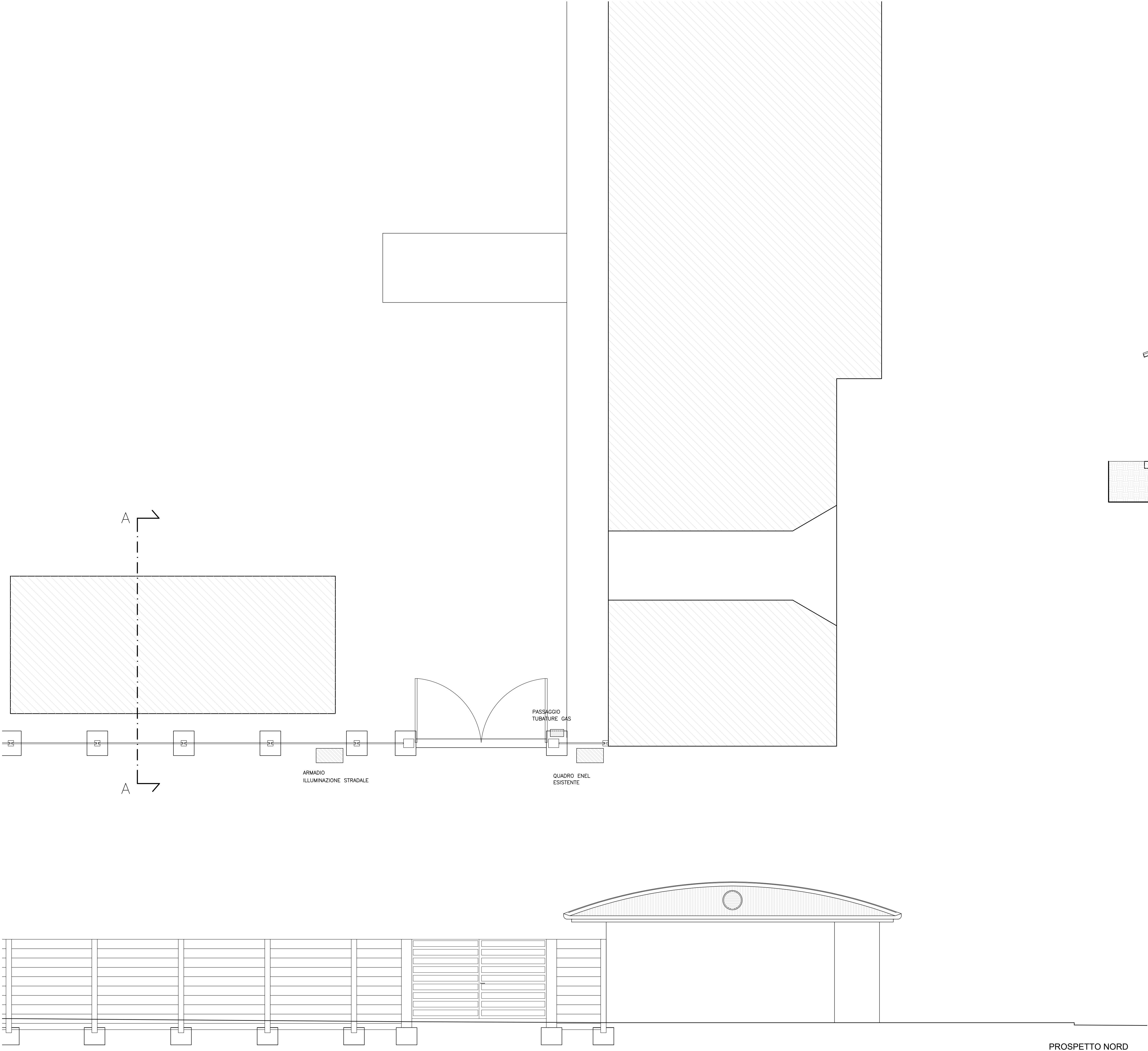
PROSPETTO NORD
